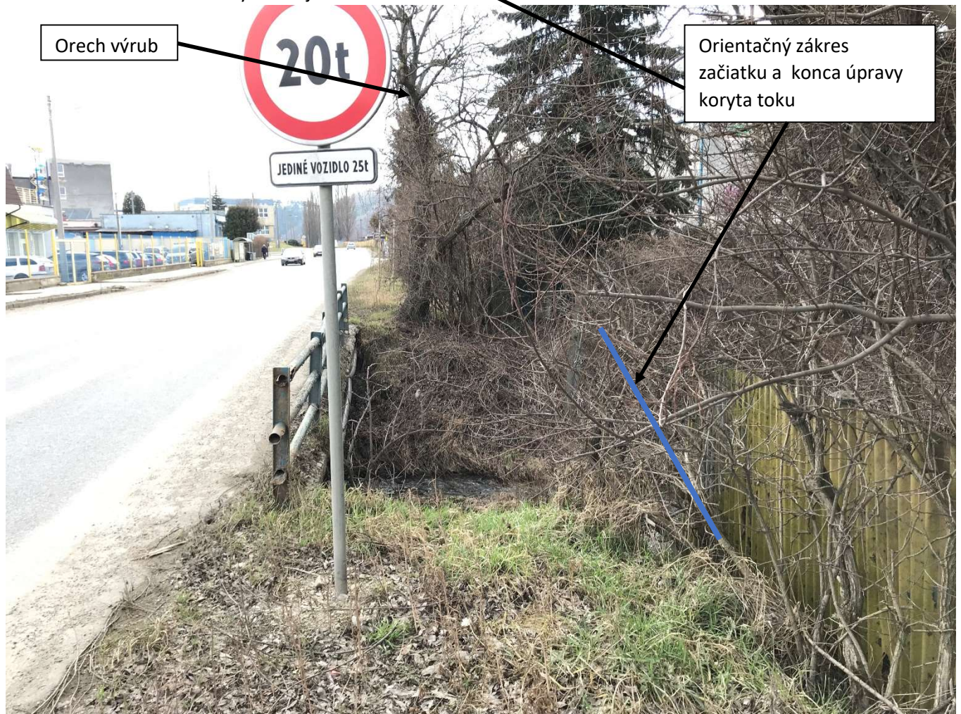
Obr. 2: Pohľad na most na výtokovej strane
